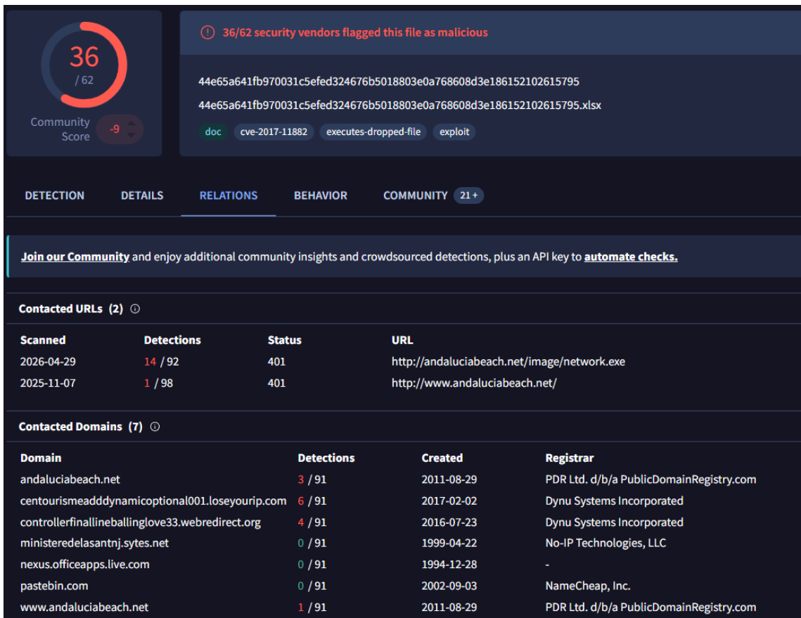
Figura 7: Clasificación del malware con detección de dominios C2.
