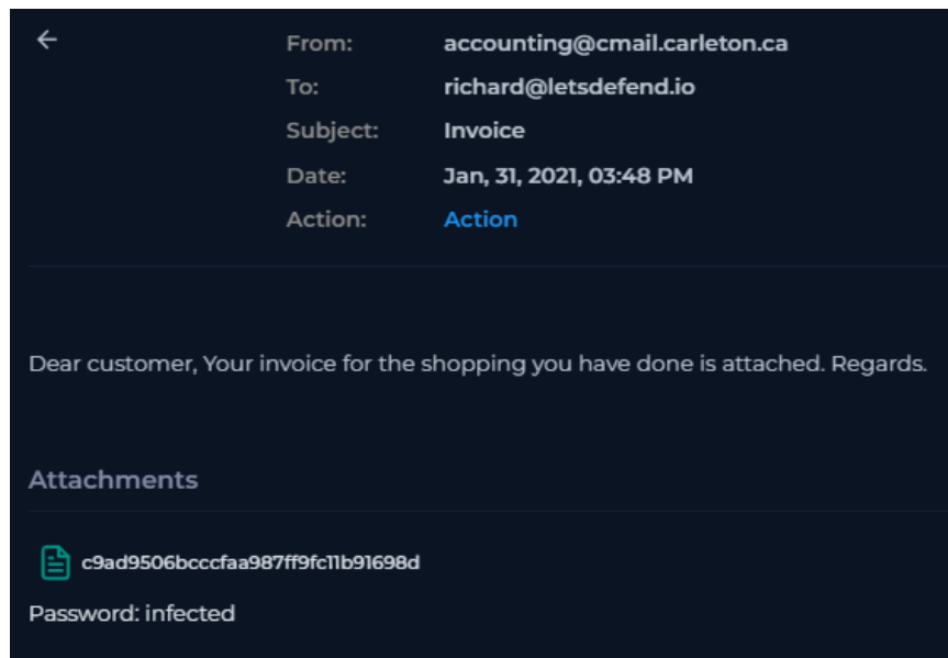
Figura 2: Revisión del contenido del correo electrónico sospechoso.
